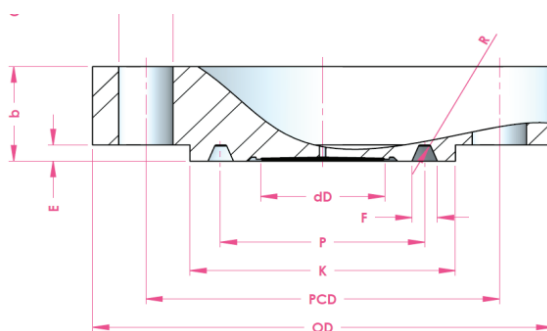
Dimensions tables
